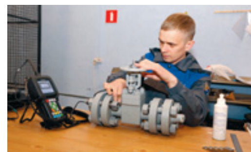
Дефектоскопист Павел Шорохов измеряет толщину металла
